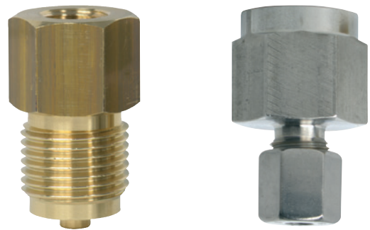
Рис. слева: Переходник наружная-внутренняя резьба, G ½ / G ¼ В Рис. справа: Компрессионный фитинг с муфтой, G ½ 400/6
